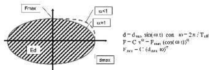
Fig. 11.9.2 – Dispositivi a comportamento viscoso
