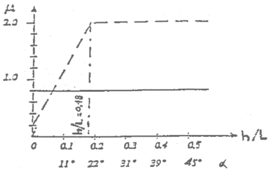
Fig. C.6.7 - Coefficienti di forma per differenti valori del rapporto freccia/luce.
